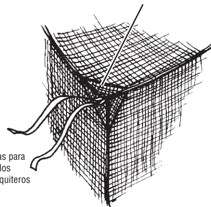
Triángulos de tela adicional para fortalecer las esquinas
